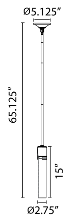
P11701 - 12" SHADE
